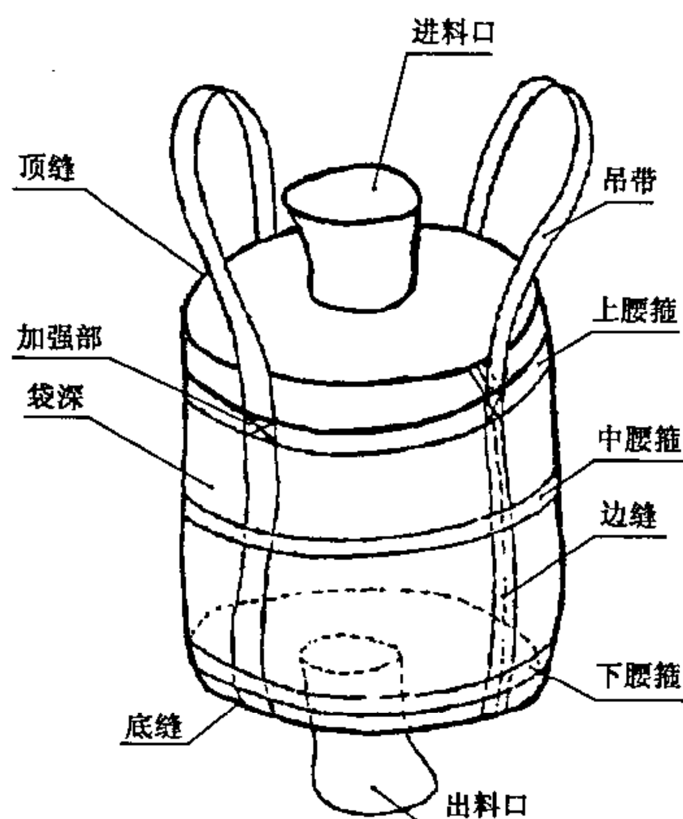
图 1 集装袋各部分结构示意图
